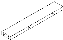
355*60*18 19 x1
